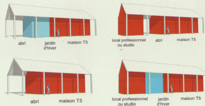
Sur une base de maison T5, croquis des diverses évolutions possibles.
